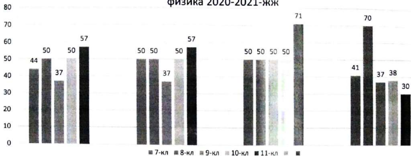
физика 2020-2021-жж
